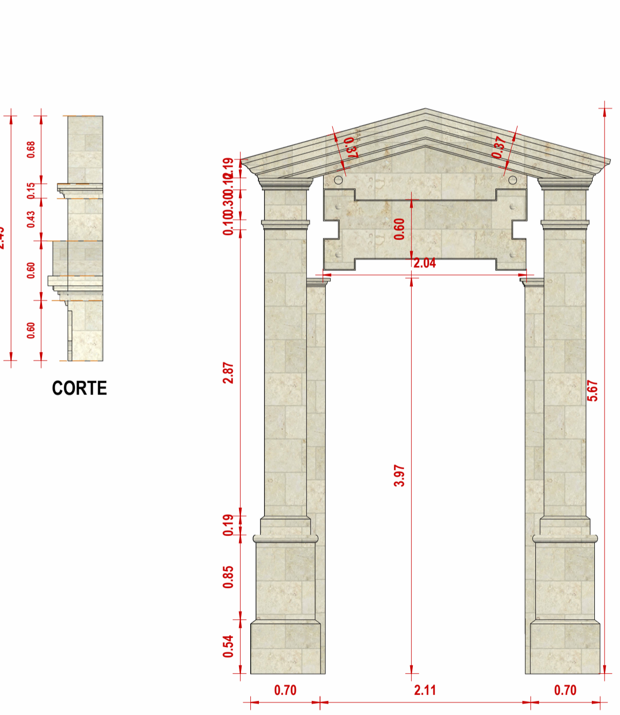
FRONTON-13 Esc. 1 : 25
