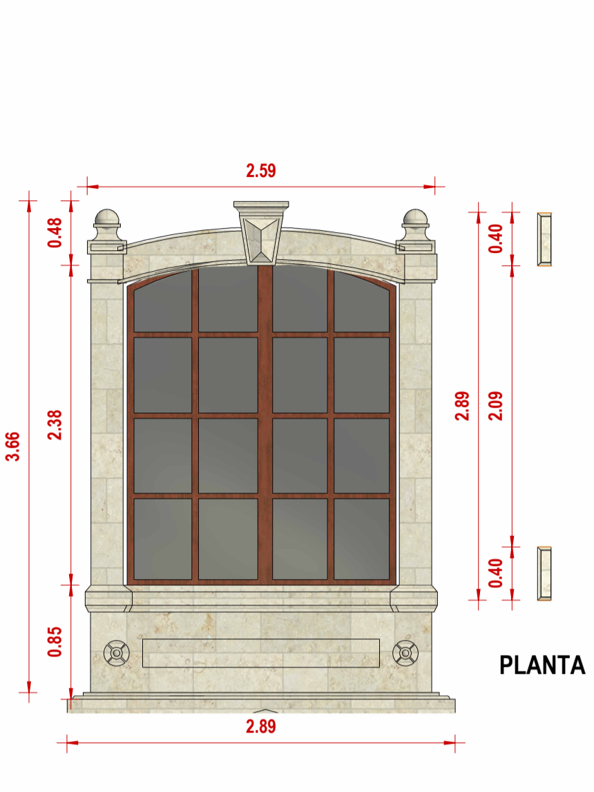
ARCO SEGMENTARIO Esc. 1 : 25
