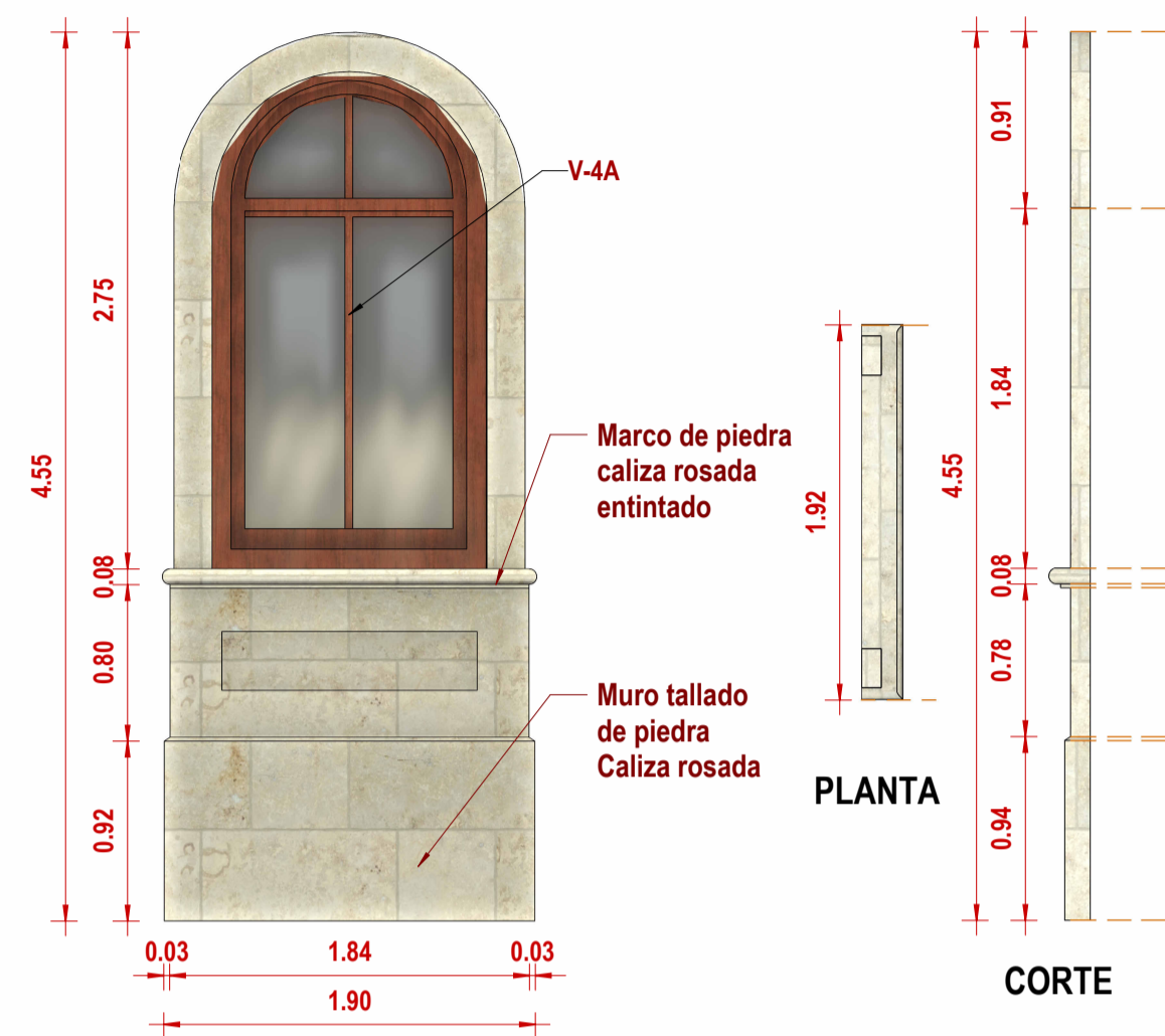
ARCO DE MEDIO PUNTO Esc. 1 : 25
