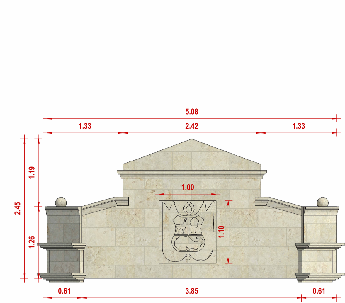
FRONTON-11 Esc. 1 : 25
