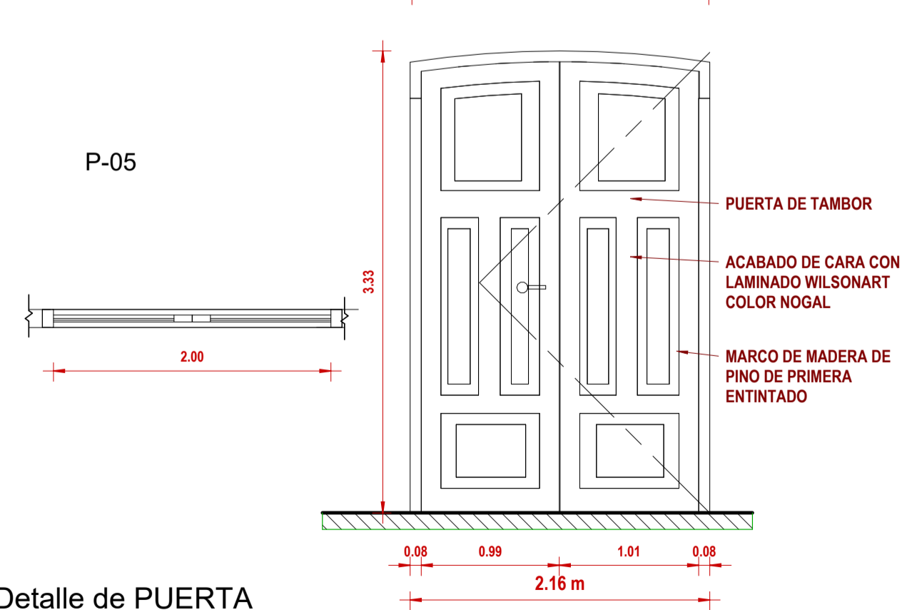
Detalle de PUERTA 1 : 25
