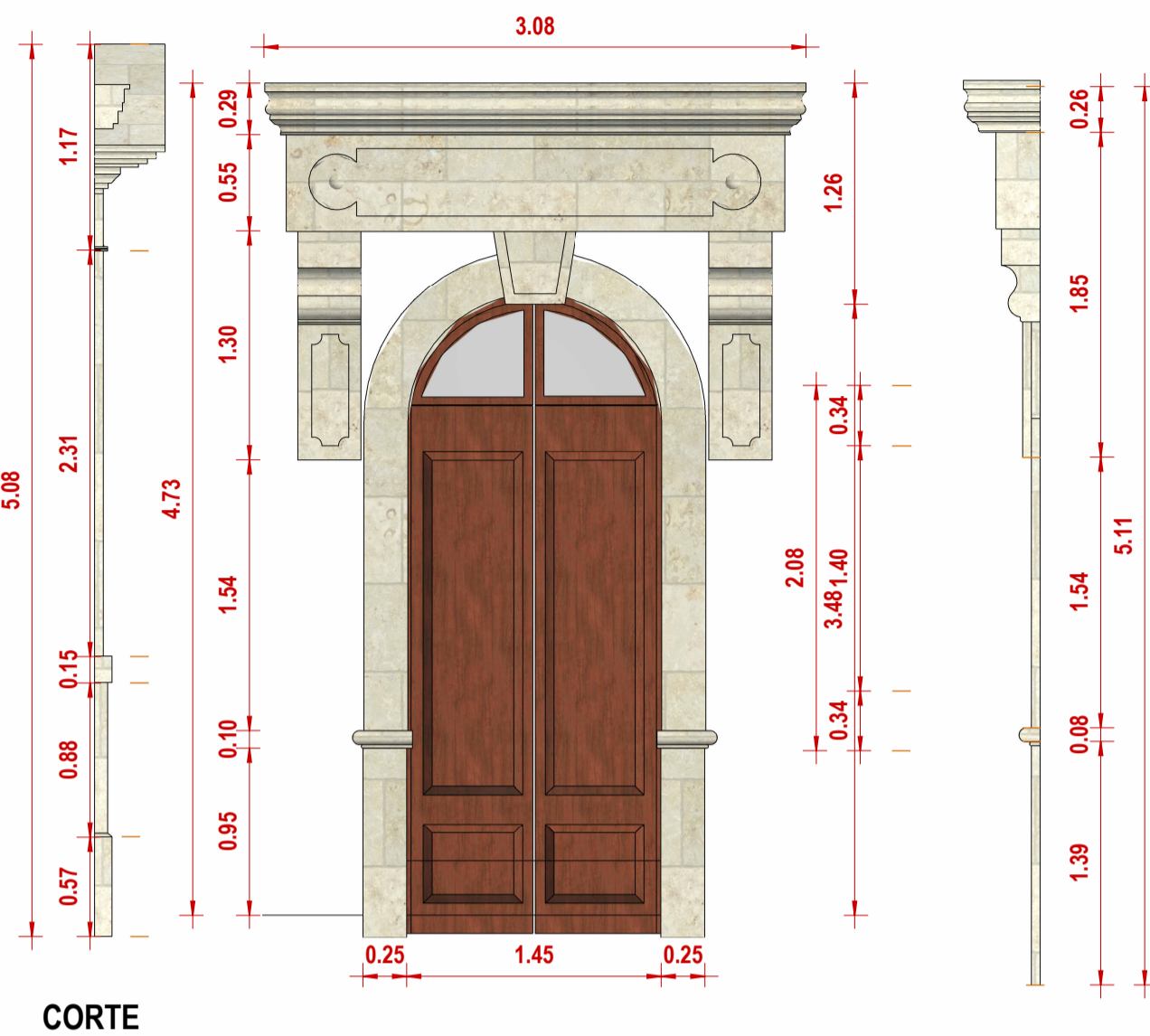
FRONTON-05 Esc. 1 : 25
