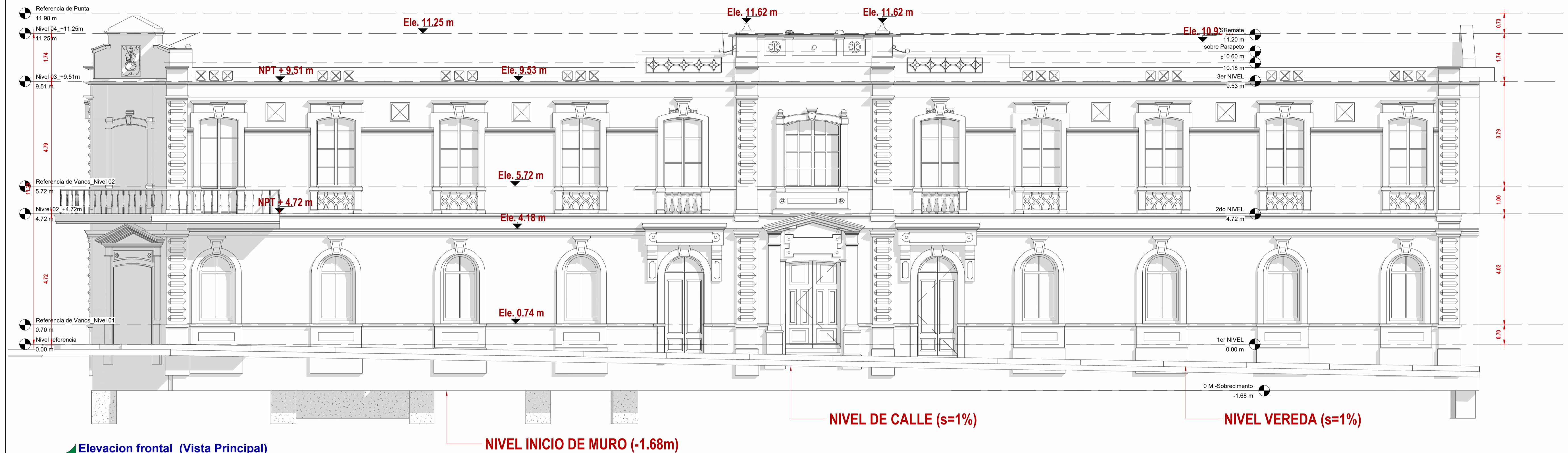
Elevacion frontal_(Vista Principal) Esc. 1 : 50
