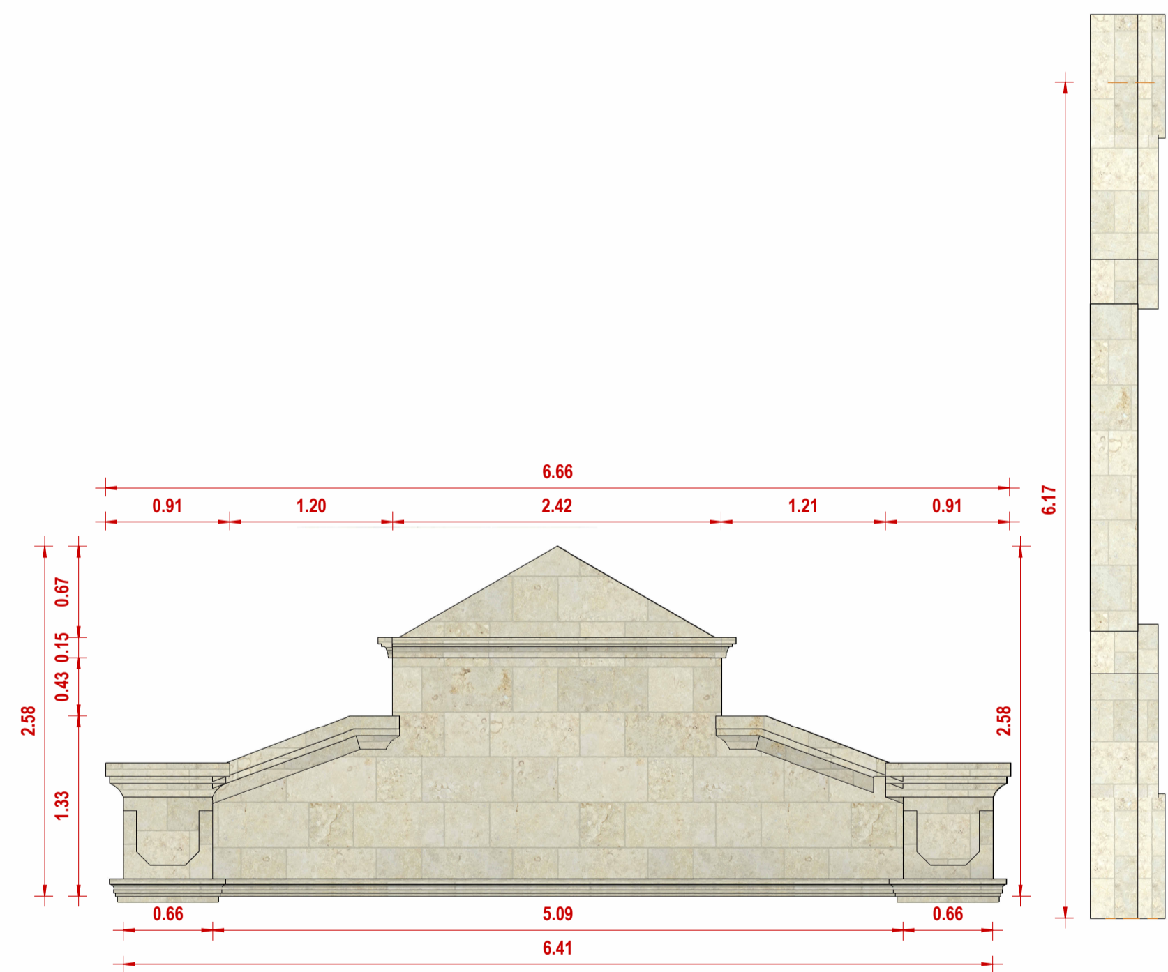
FRONTON-12 Esc. 1 : 25
