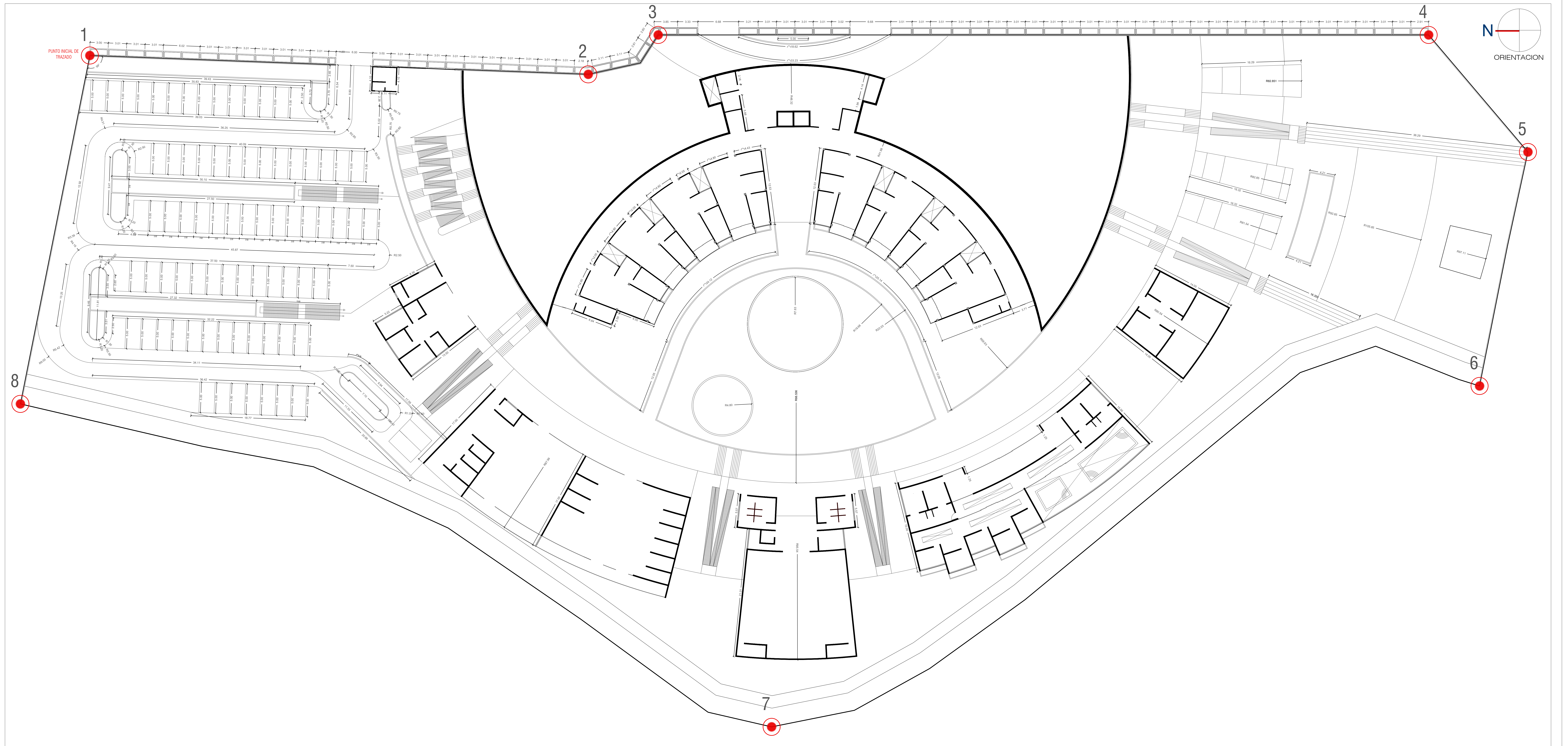
PLANIMETRIA GENERAL TRAZADO ESCALA 1:200
